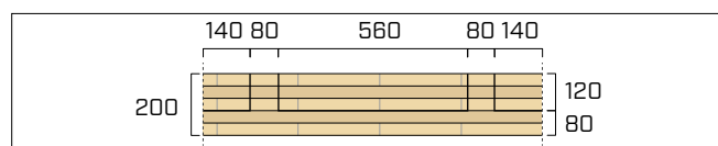
geometrie frézování
