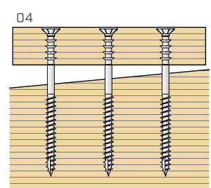
Reglați în același mod și celelalte șuruburi pentru a echilibra structura.
