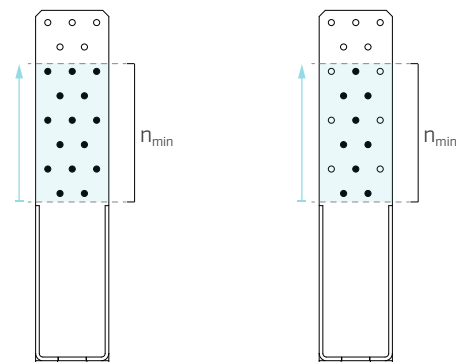
WHT20: fixare parțială în configurația wide pattern și respectiv narrow pattern, cu instalarea numărului minim de conectori n_{\min} .
